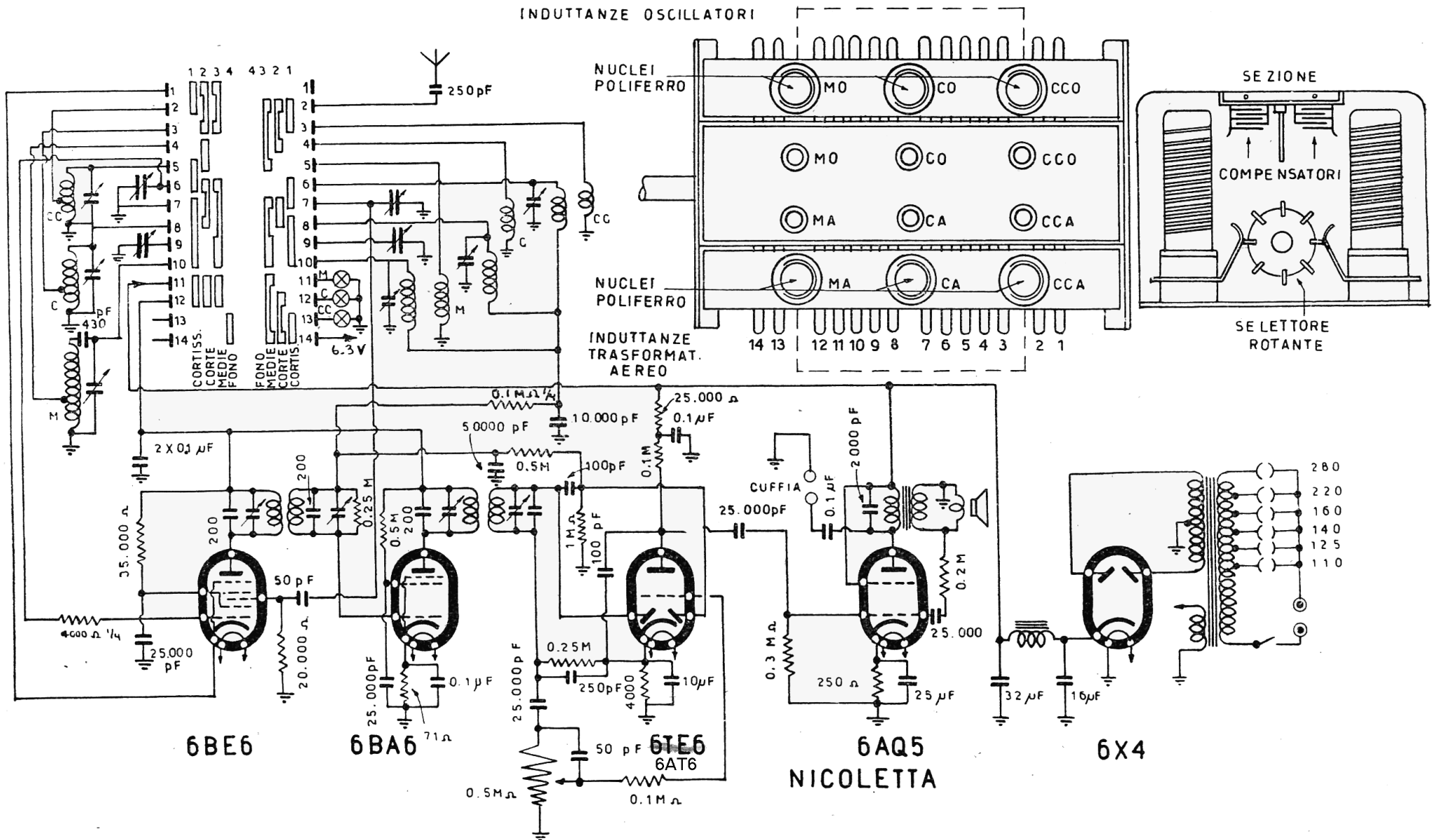
INCARADIO - Mod. IF 51 « NICOLETTA ». Gamma onde medie intera, gamma onde corte-cortissime da 13 a 51 metri, con allargamento di banda continuo, mediante condensatore variabile e comando sintonia separati. Media frequenza 460 kc. Altoparlante a magnete permanente. Potenza d'uscita 4 watt.
